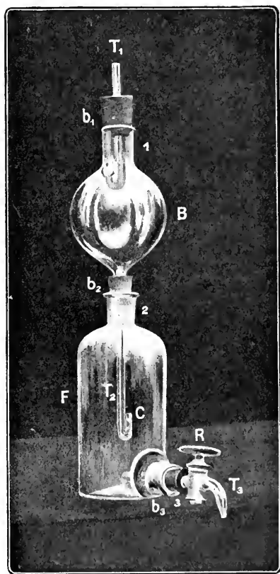
FIG. 236.—Radiogenic. (Siemens.)
